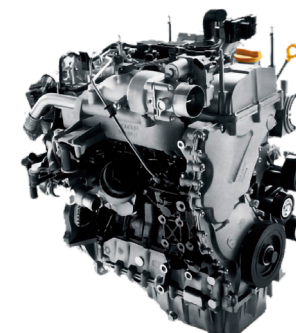
Motor Turbodiésel Inyección Directa Cilindrada (cm³): 1.996 / 4 cilindros Potencia (kW (CV)/rpm): 108,5 (150) / 3.500
