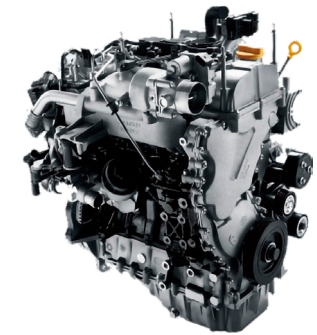
Motor Turbodiésel Inyección Directa Cilindrada (cm 3 ): 1.996 / 4 cilindros Potencia (kW (CV)/rpm): 108,5 (150) / 3.500
